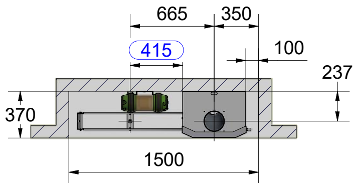
K-K ( 1 : 30 )
