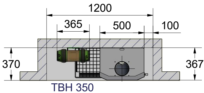
D-D ( 1 : 25 )
