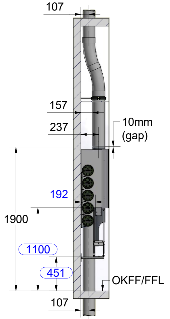
L-L ( 1 : 30 )
