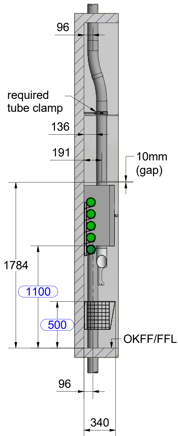
E-E ( 1 : 25 )
