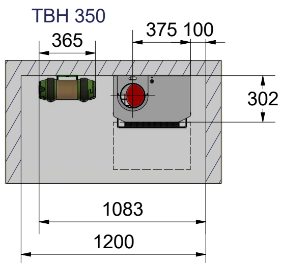
A-A ( 1 : 25 )
