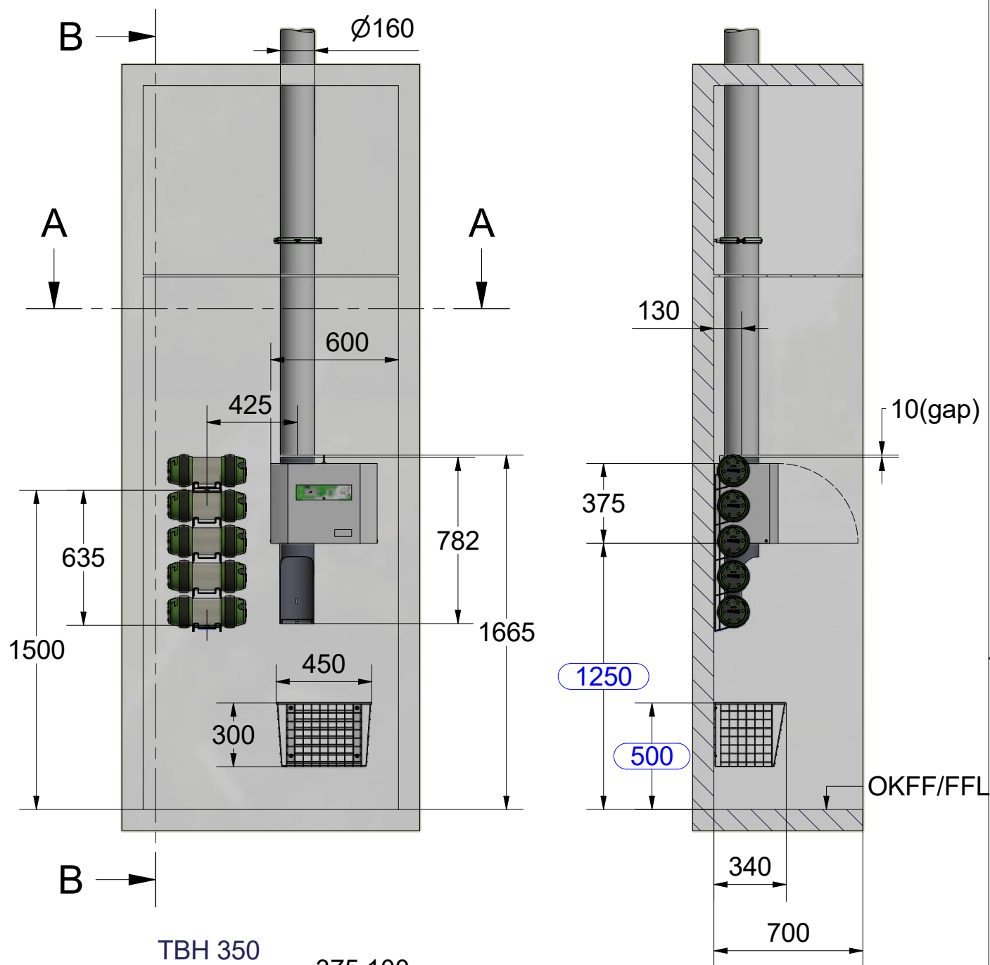
B-B ( 1 : 25 )
